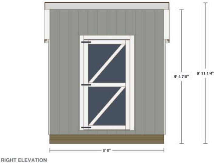
RIGHT ELEVATION
