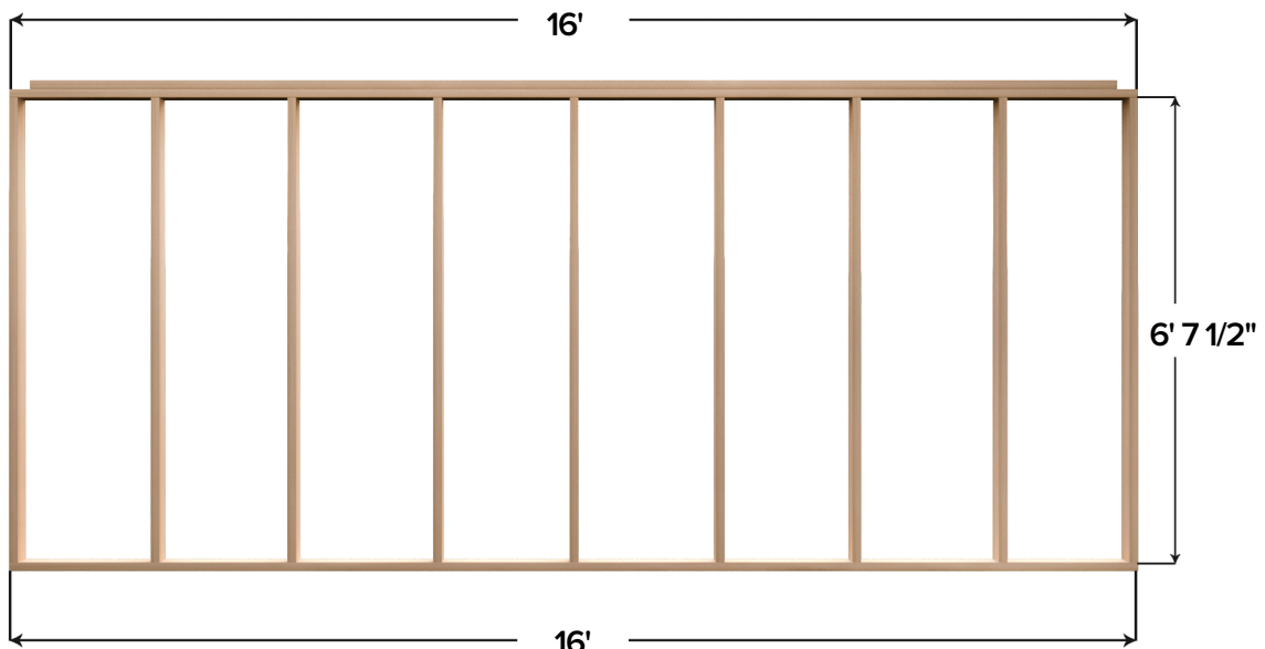
LEFT WALL
