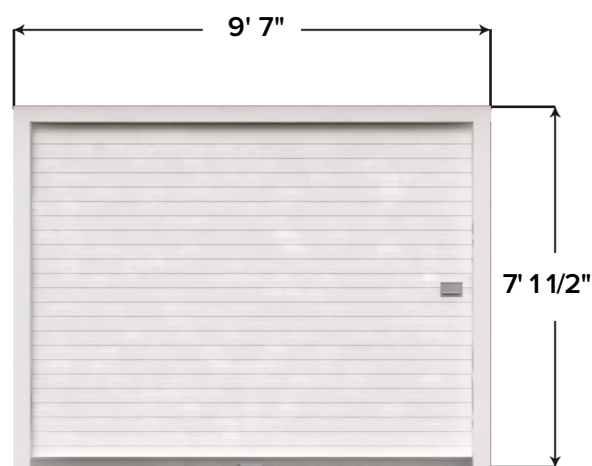
DOOR
