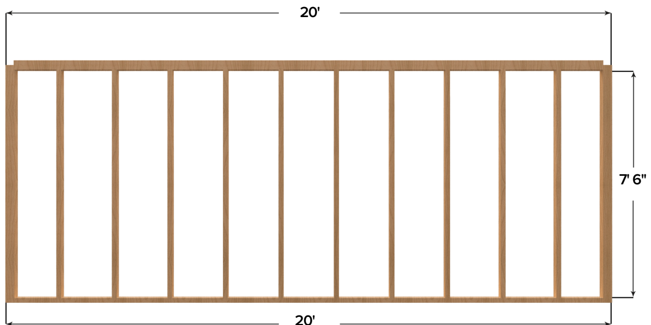
LEFT WALL
