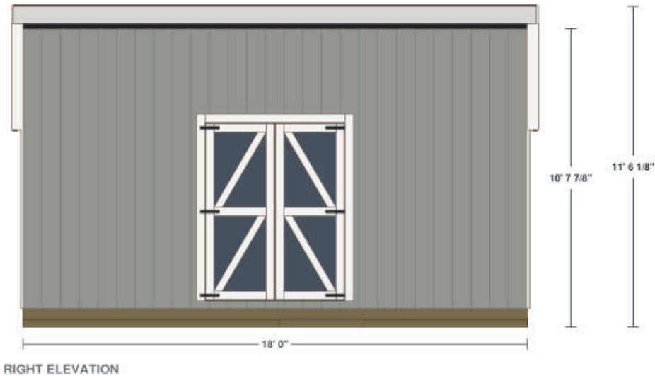
RIGHT ELEVATION
