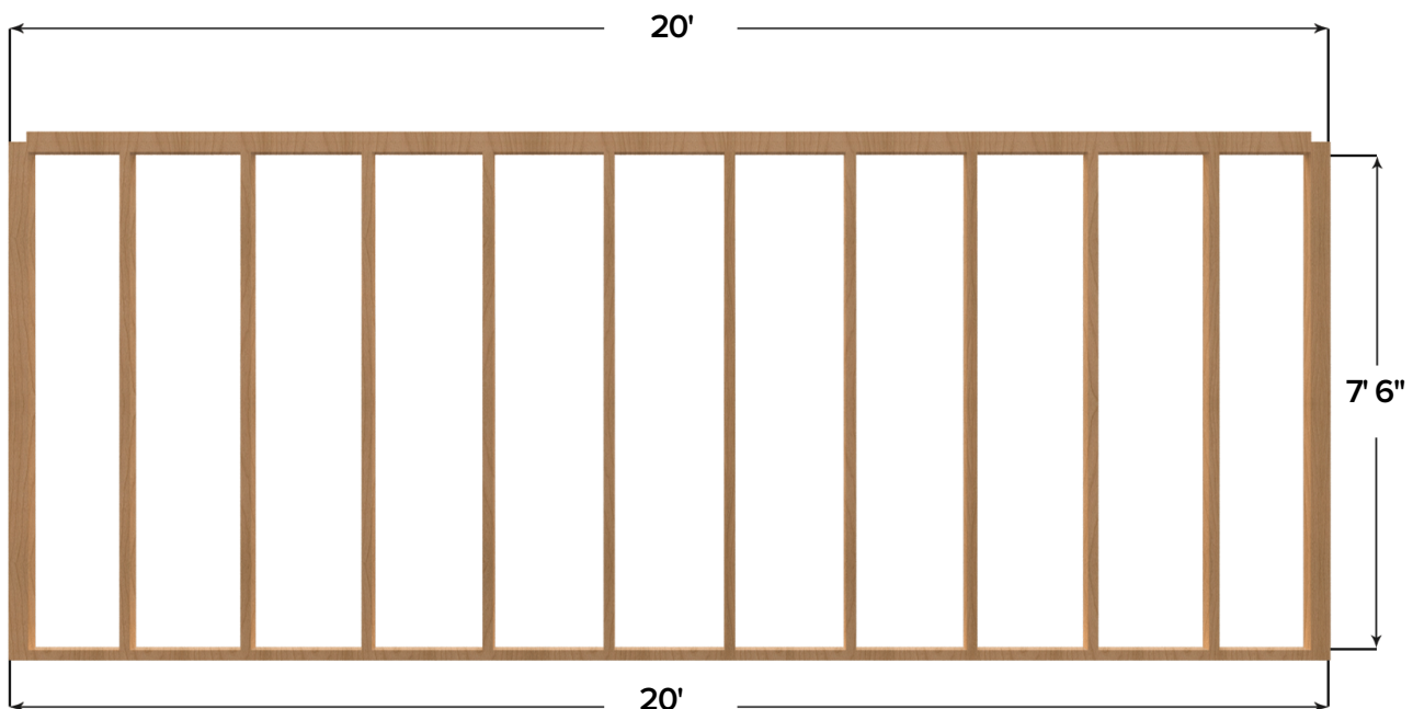
LEFT WALL
