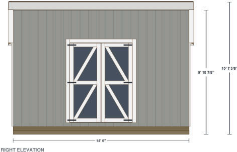
RIGHT ELEVATION
